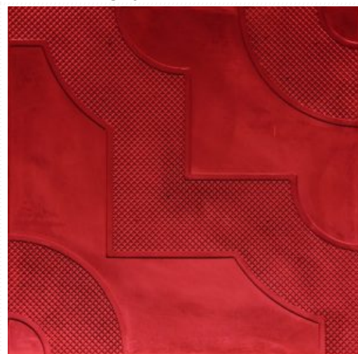
قالب وکیوم گلبرگ 40X40X3.5
